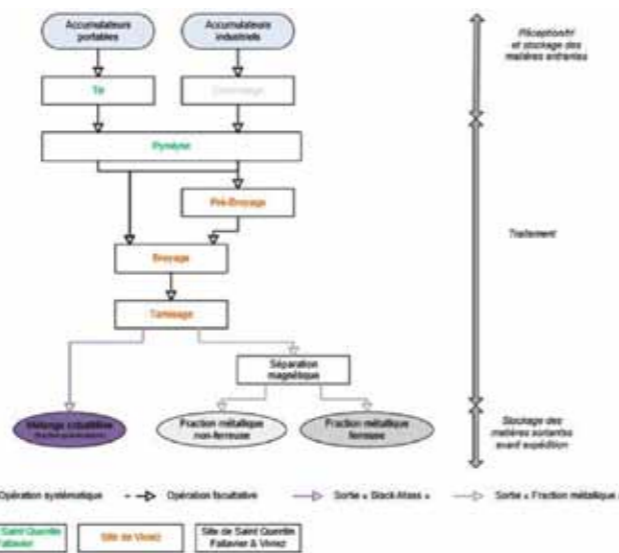
Processus schématique de recyclage des accumulateurs portables et accumulateurs industriels par la société SNAM
